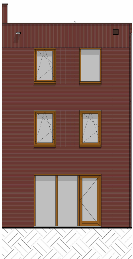
achtergevel 1 : 100
