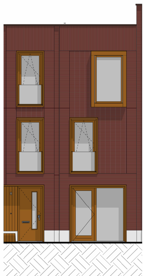
voorgevel 1 : 100
