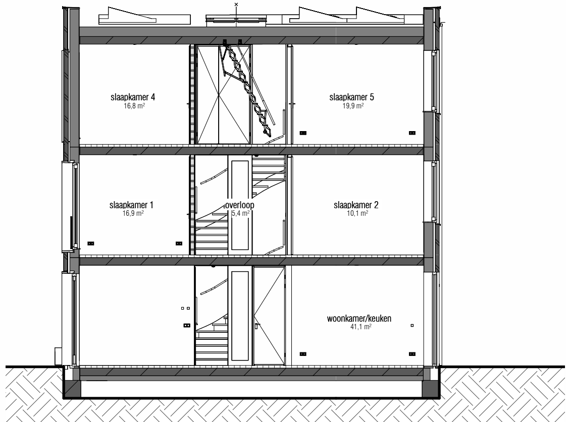
doorsnede 1 : 100
